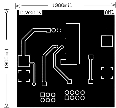
Figure 5e. Bottom Layer
